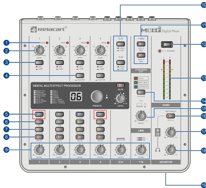
MiXX8.6 (调音台) 前面板
